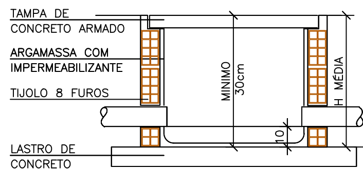
Detalhe – Caixas de Inspeção tipo 1 escala —————+ 1/20
